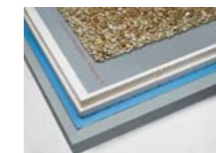
Свободная укладка с балластом
